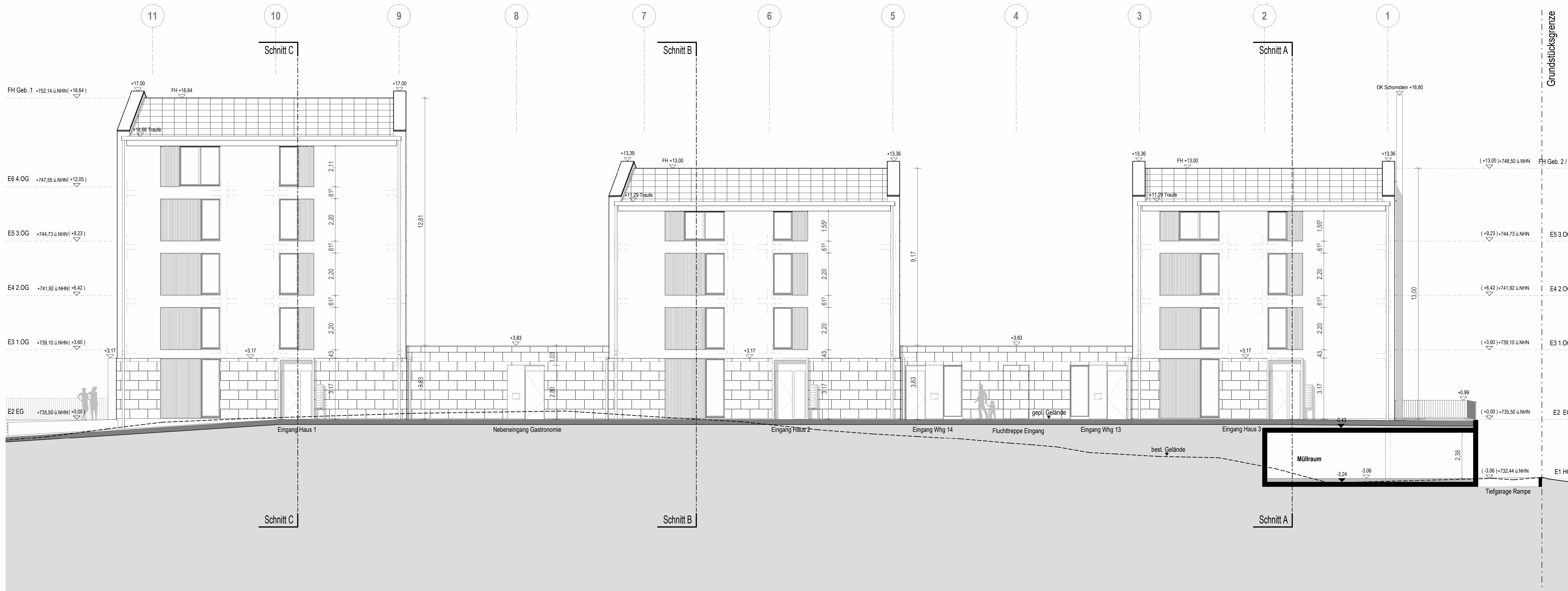
Ansicht Ost
